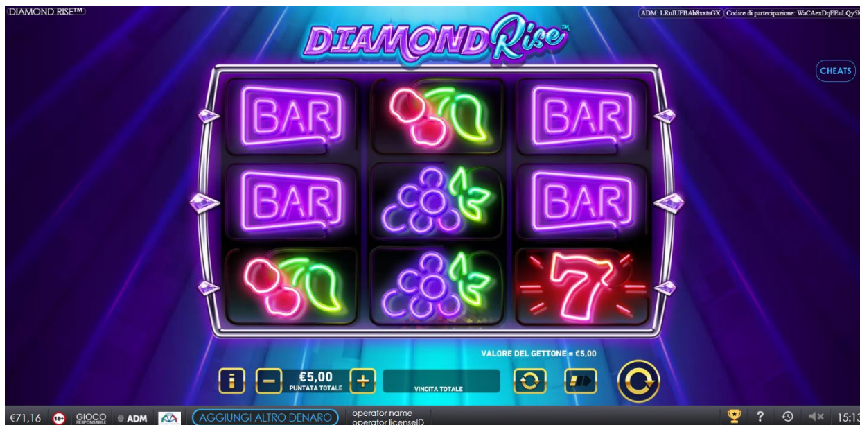
Schermata principale
